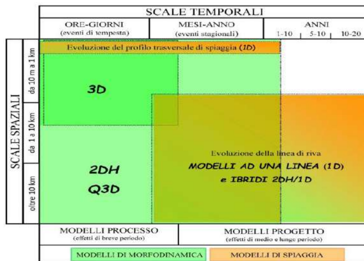
Figura 9 - Schematizzazione della diversa tipologia dei modelli di trasporto utilizzabili in relazione al variare delle scale spaziali e temporali. Lisi et al. (2017)
