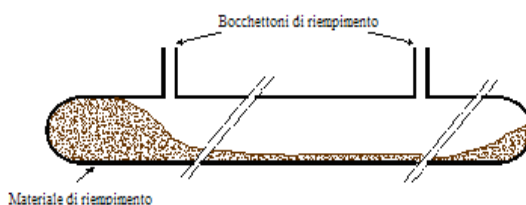
Figura 13 - sezione longitudinale del geotubo
