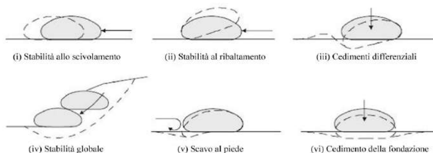
Figura 18 - geotubi: stati limite esterni (Lawson 2006)
