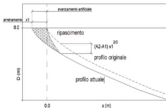
Figura 11 - ripascimento con sedimenti di granulometria molto maggiore di quelli presenti in sito (Noli 2005)
