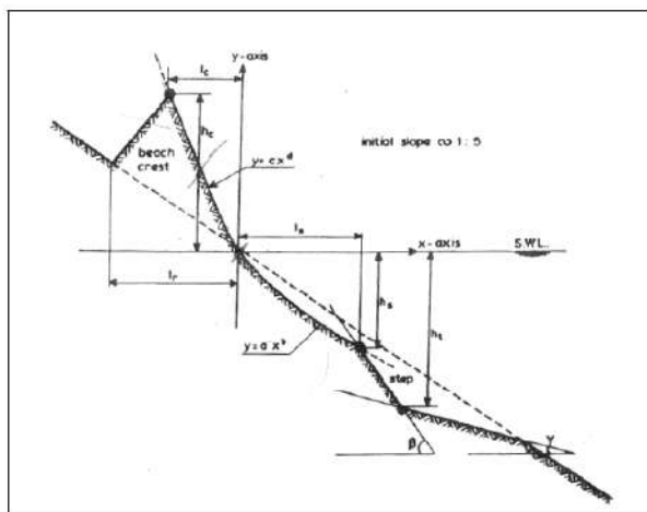
Figura 12 - profilo di spiaggia di ghiaia (Van der Meer 1988)
