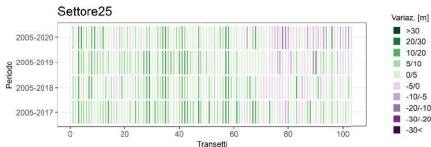
Figura 4 - Evoluzione di dettaglio della linea di riva del settore 25 (Foce Fosso ai Molini – La Riconiata) a nord di San Vincenzo (LI), globalmente stabile ma caratterizzato da porzioni con tendenze opposte nel periodo di osservazione (RT-LaMMA, 2021)
