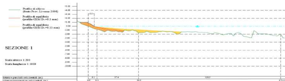
Figura 10 - esempio di profilo intersecante di tipo a): confronto tra due materiali di ripascimento con diversa granulometria, a parità di avanzamento atteso della linea di riva.
