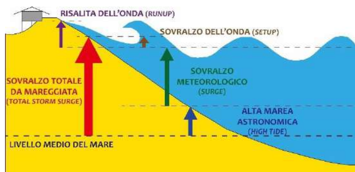
Figura 6 - Schema dei principali fattori che caratterizzano le mareggiate (Regione Emilia Romagna 2020)
