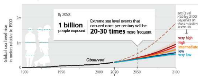
Figura 7 - innalzamento del livello medio del mare in relazione al 1900 , IPCC, 2023
