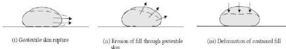
Figura 19 - geotubi: stati limite interni (Lawson 2006)
