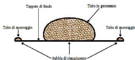
Figura 14 - sezione trasversale del geotubo
