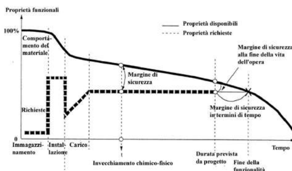
Figura 17 – Andamento delle proprietà richieste e disponibili in funzione del tempo (da ISO Technical Report 13434)
