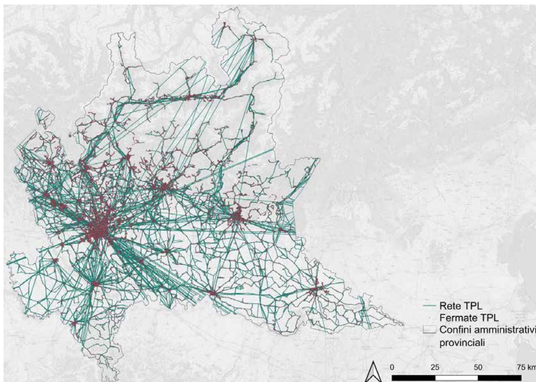
Figura 3 - Rete e fermate TPL
